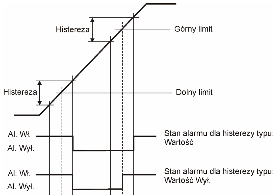
Rys. 1 Schemat działania alarmu typu Zakres Wył.
